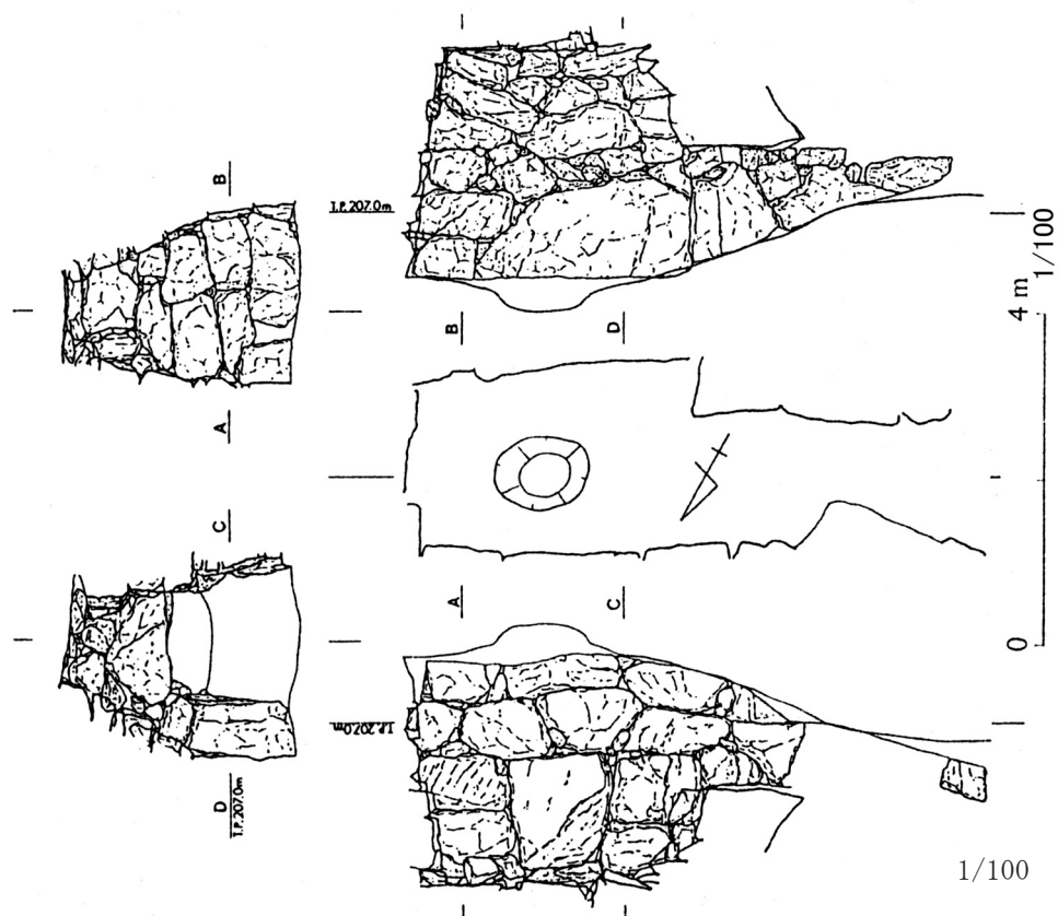
図 188 稻荷神社裏山1号墳横穴式石室実測図
