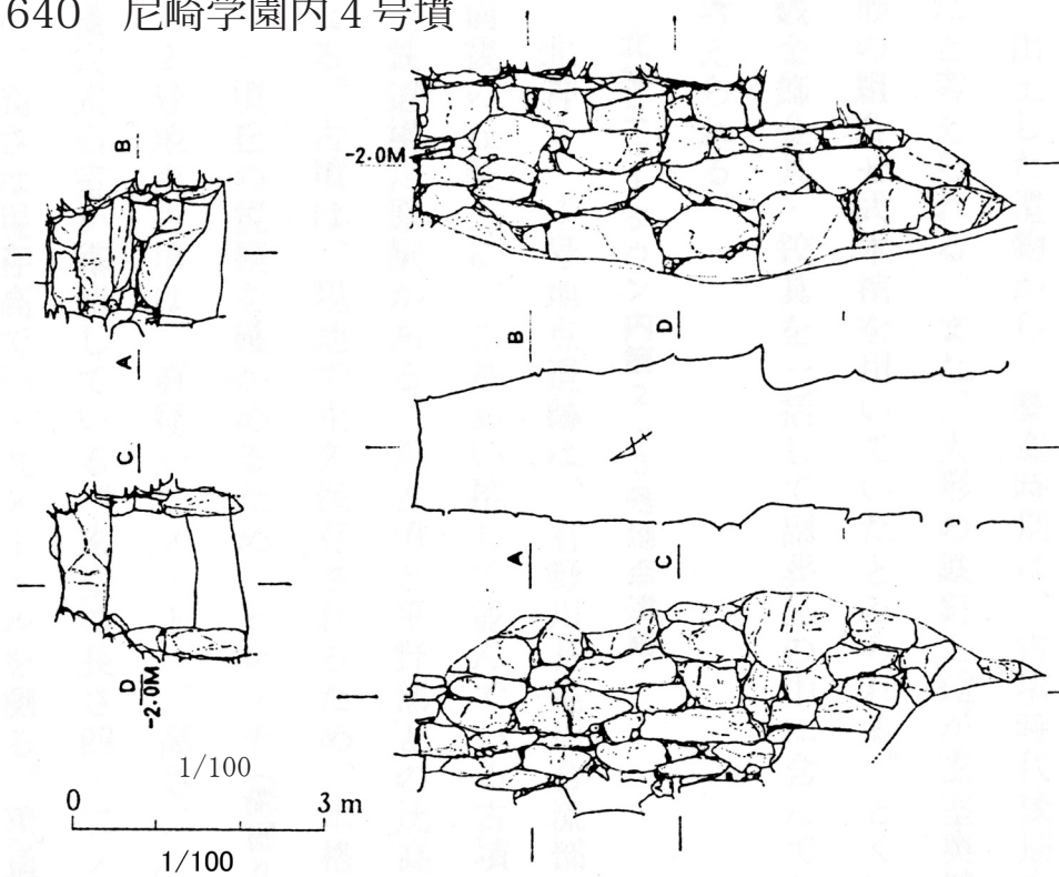
図 189 尼崎学園内4号墳石室実測図
