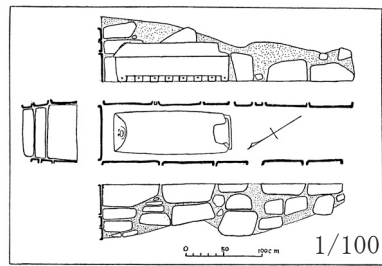
第3図 石室および陶棺置状況実測図
