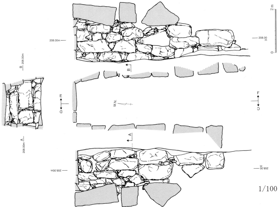
第3図 北ノ脇古墳群第2号墳石室実測図
