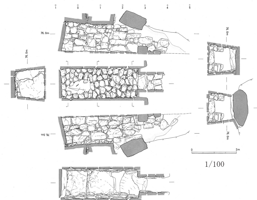
第6図 石室実測図
