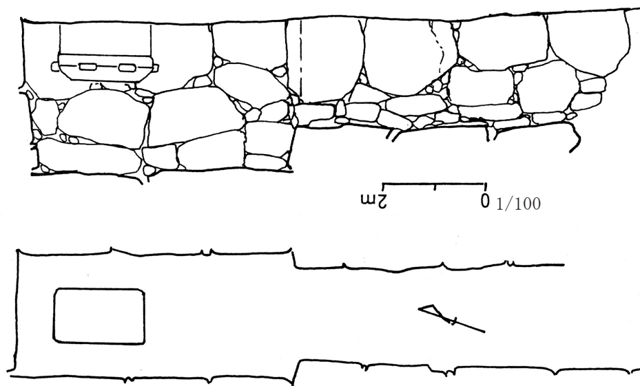
付図2 中山寺白鳥塚古墳石室実測図
