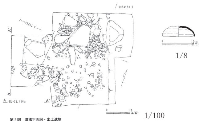
第2図 遺構平面図・出土遺物
