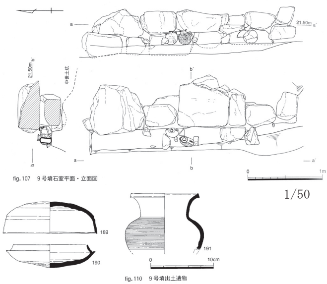
fig.110 9号墳出土遺物
