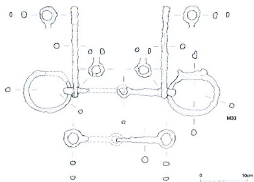
第28図 13号墳出土鉄器
