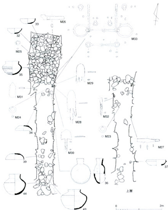
第26図 13号墳石室遺物出土位置
