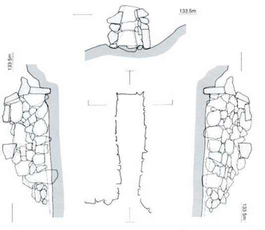
第50图 28号墳石室平面図・立面図 1/100
