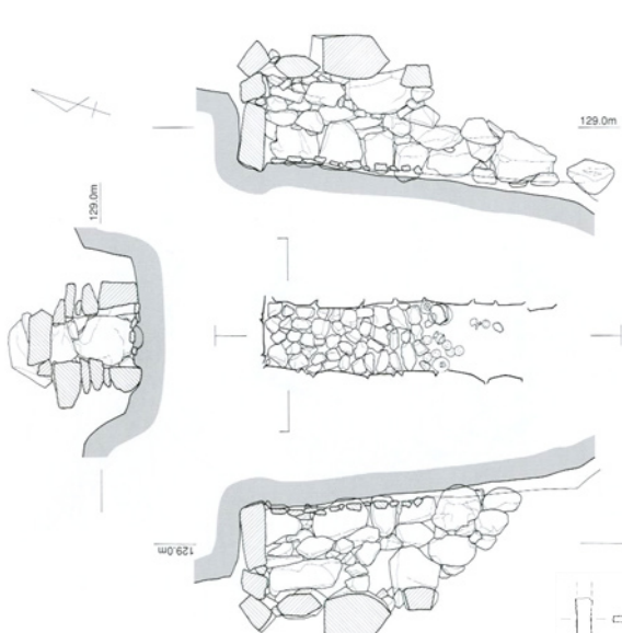
第42图 27号墳石室平面図・立面図 1/100
