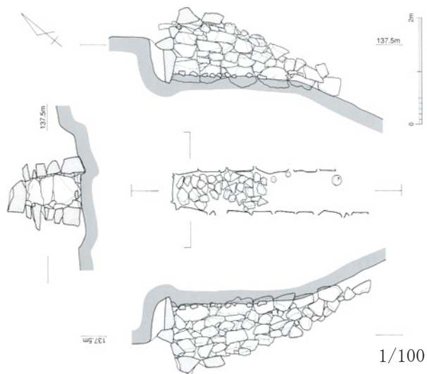
第59図 29号墳石室平面図・立面図
